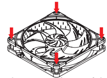
Charge de compression maxi de 7,5 Kg par vis (total de 30 Kg)
